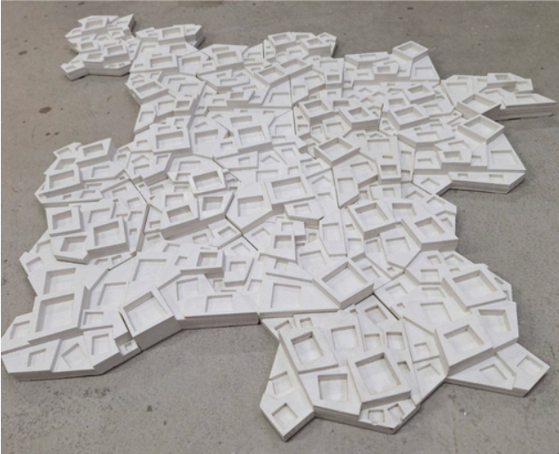
Antropoceno
